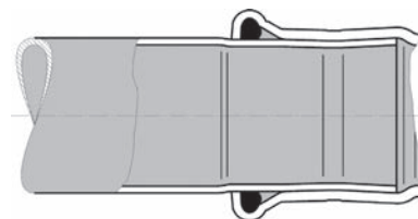
Bild 4: Verpressung der Abmessungen 76,1 mm bis 108 mm in 2 Ebenen
