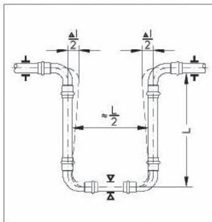
Bild 8: U-Rohr-Kompensator
