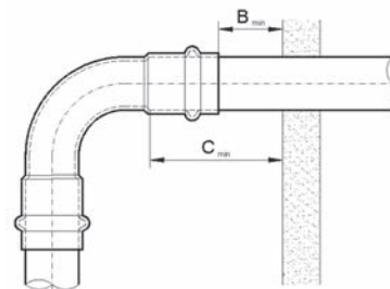
Bild 13: Mindestabstand zwischen Wand und Pressstelle
