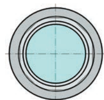
Bild 3: 8-Kant-Verpressung bei Abmessungen bis 35 mm, annähernd rundes Pressbild
