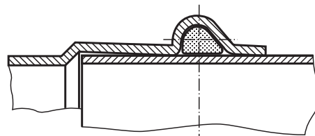
Bild 2: Rohrverbindung verpresst, Abmessungen bis 42 mm
