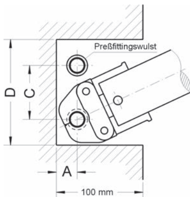
Bild 16: Mindestbreite D von Nischen, Mindestabstand A der Leitungen zur Nischenrückwand und Mindestabstand C der Leitungen untereinander
