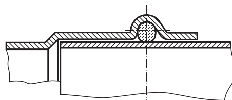
Bild 1: Rohrverbindung unverpresst, Abmessungen bis 42 mm
